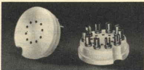
Per semplificare il montaggio si può usare questo tipo di zoccolo a pressione inserendo in esso il circuito integrato come se fosse un transistor.
