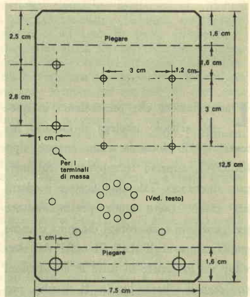
Fig. 2 - Il circuito completo, comprese le pile d'alimentazione, può essere montato su una piccola piastra d'alluminio da 7,5 x 12,5 cm, forata e piegata per formare un telaio di supporto.
