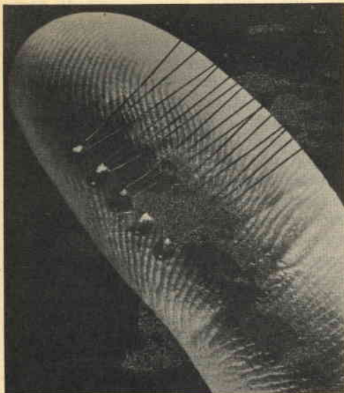
Fig. 5 - Nuova serie di transistori microminiatura ad alte prestazioni incapsulati in plastica, prodotti dalla General Electric Company (USA).
